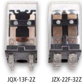
JQX-13F-2Z JZX-22F-3Z
